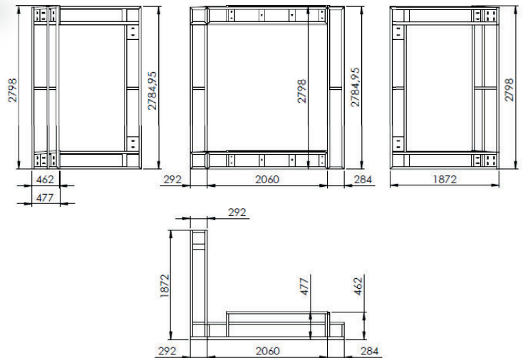
Ossature B2 (encadrement latéral) tube 40x40x2 et 80x40x2
