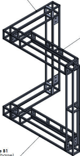
Ossature B1 (poutre haute) tube 40x40x3
